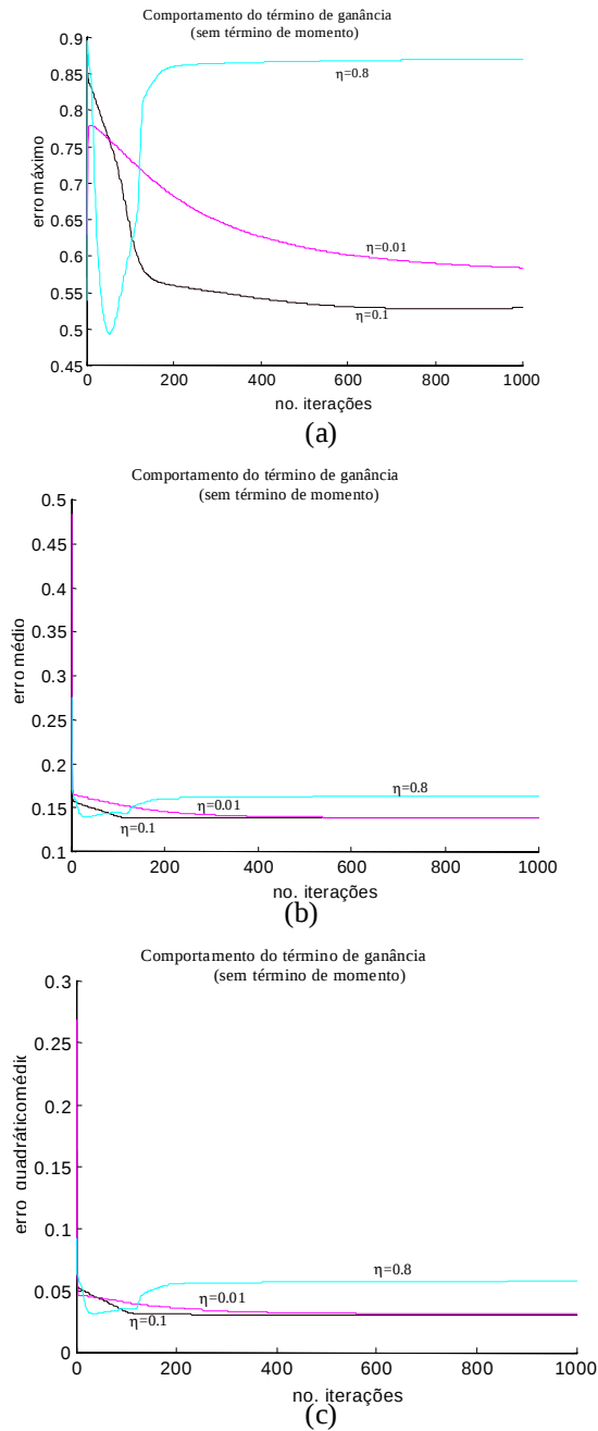
Figura 13. Comportamiento del término de ganancia, sin término de momento, respecto a los errores.
