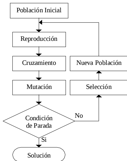
Figura 1. Principio de funcionamiento de un GA.
