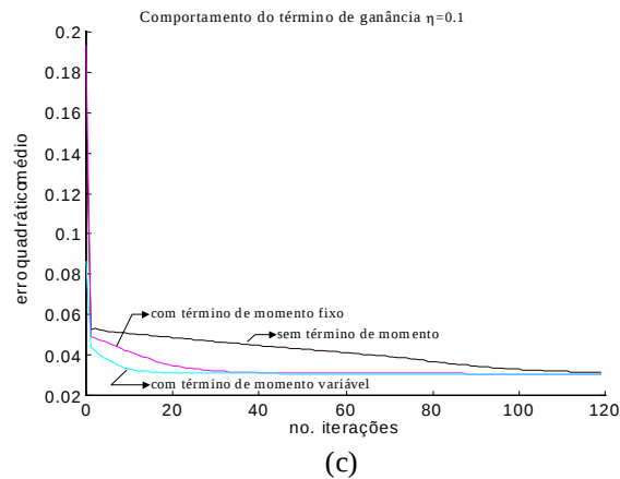
Figura 16. Comportamento del término de ganancia \eta=0.1 , con los diferentes términos de momentos, respecto a los errores.
