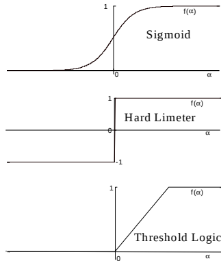
Figura 7. No-linearidades más utilizadas en Redes Neuronales.
