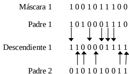
Figura 4. Cruzamiento uniforme.
