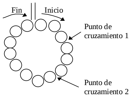
Figura 3. Cruzamiento con dos puntos.
