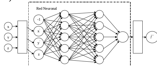
Figura 9. Estructura de la Red Neuronal empleada.
